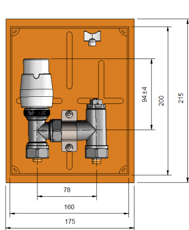
c) Wersja kasetowa „LimitBox”
